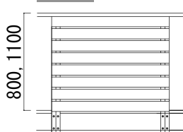
横棧
